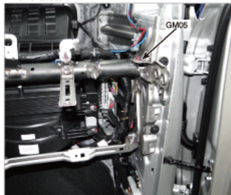
88.仪表板右侧
