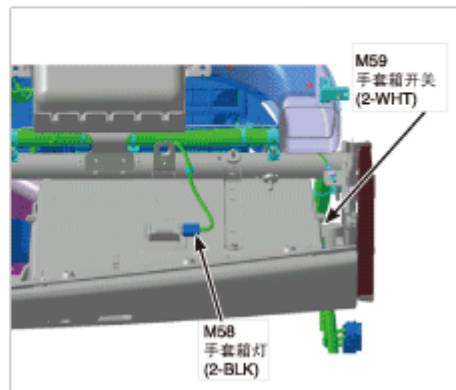
87.仪表板右侧
